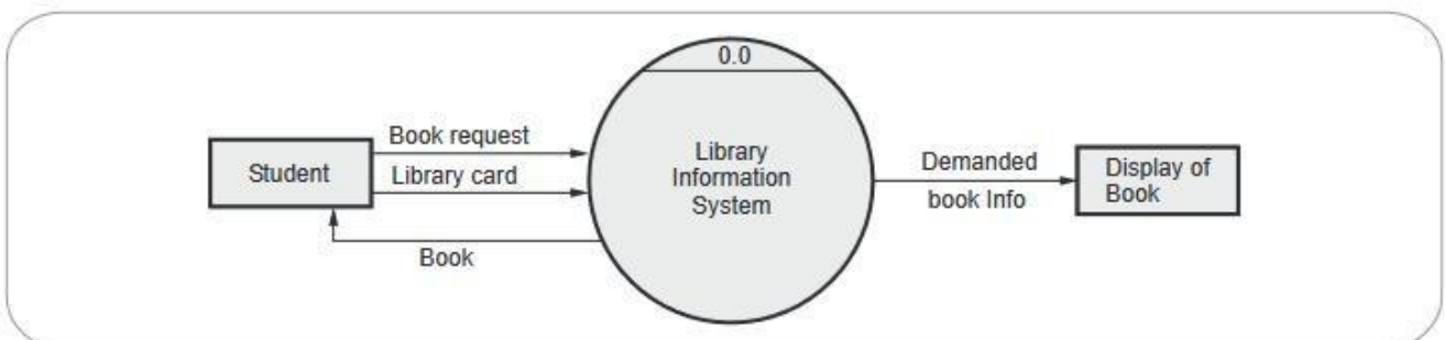
Fig. 3.4.8 Level 0 DFD (Context level DFD)
