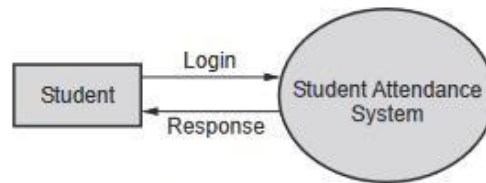
Fig. 1 Level 0 DFD
