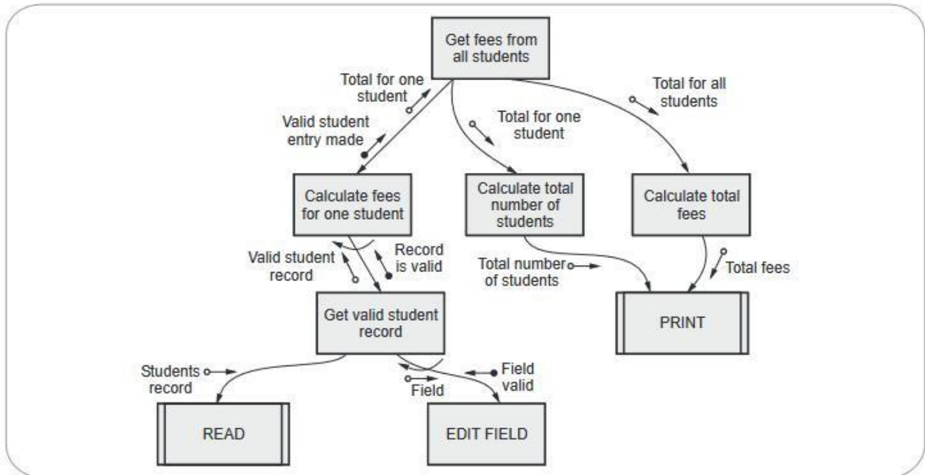
Fig. 3.4.19 Structure chart
