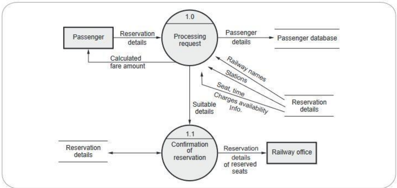
Fig. 3.4.13 Level 1 DFD
