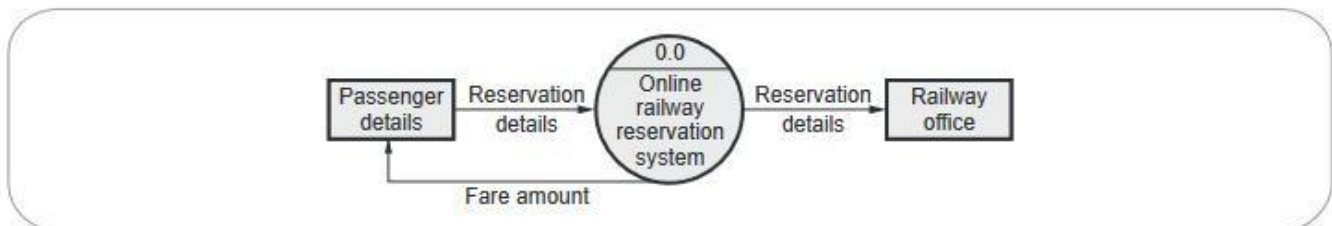
Fig. 3.4.12 Level 0 DFD
