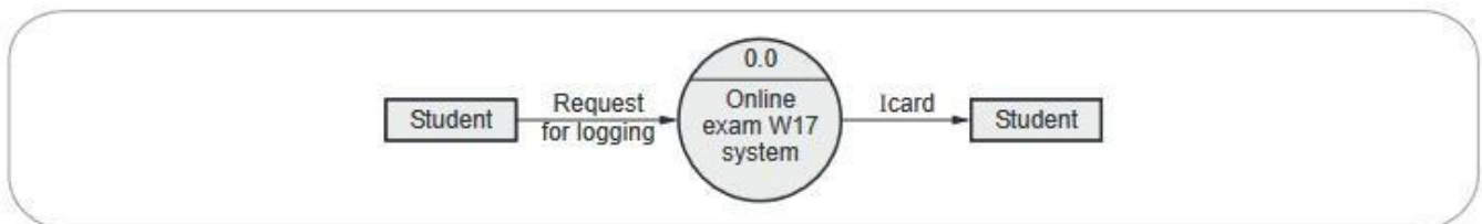
Fig. 3.4.10 Level 0 DFD
