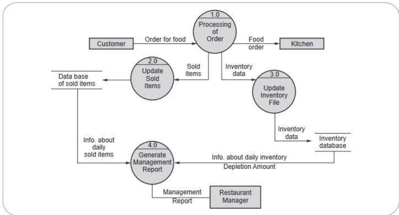
Fig. 3.4.7 Level 1 DFD
