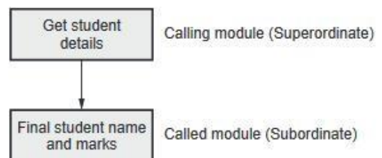
Fig. 3.4.16 Connector
