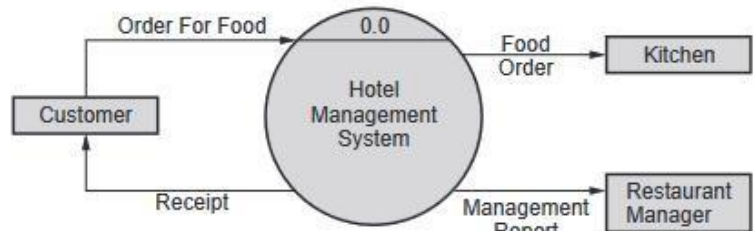
Fig. 3.4.6 Level 0 DFD
