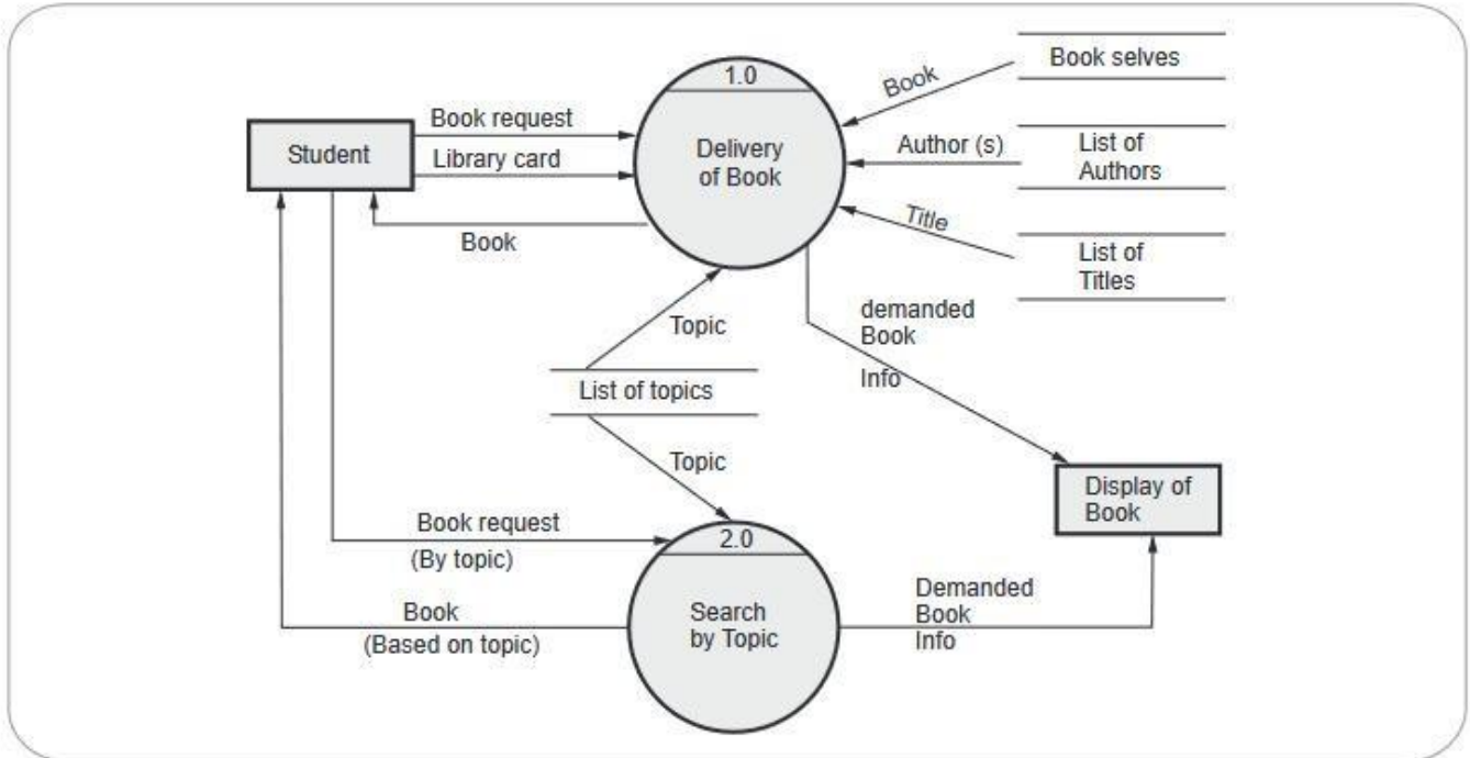
Fig. 3.4.9 Level 1 DFD
