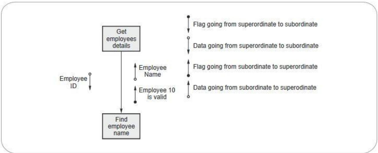
Fig. 3.4.17 Use of flag
