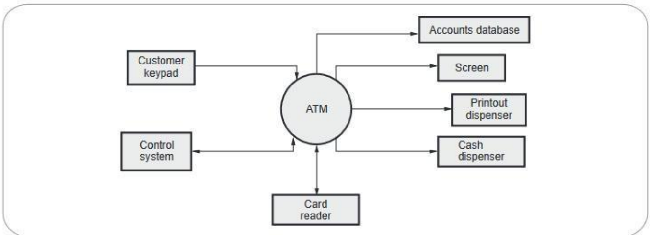
Fig. 3.4.14 Level 0 DFD
