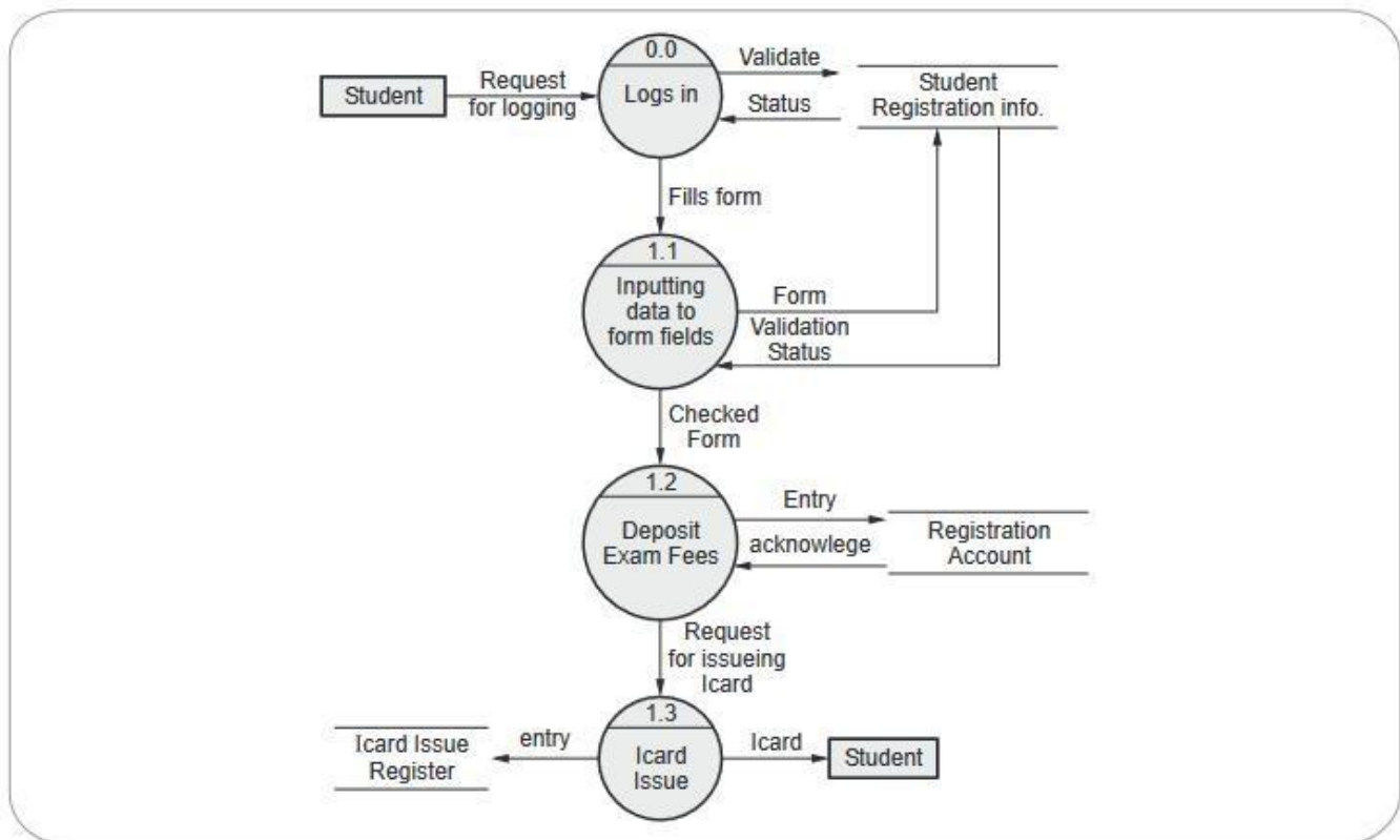
Fig. 3.4.11 Level 1 DFD
