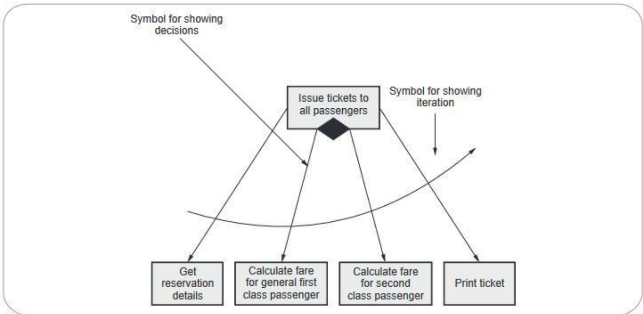
Fig. 3.4.18 Interaction
