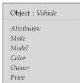
Fig. 3.1.2 Object
