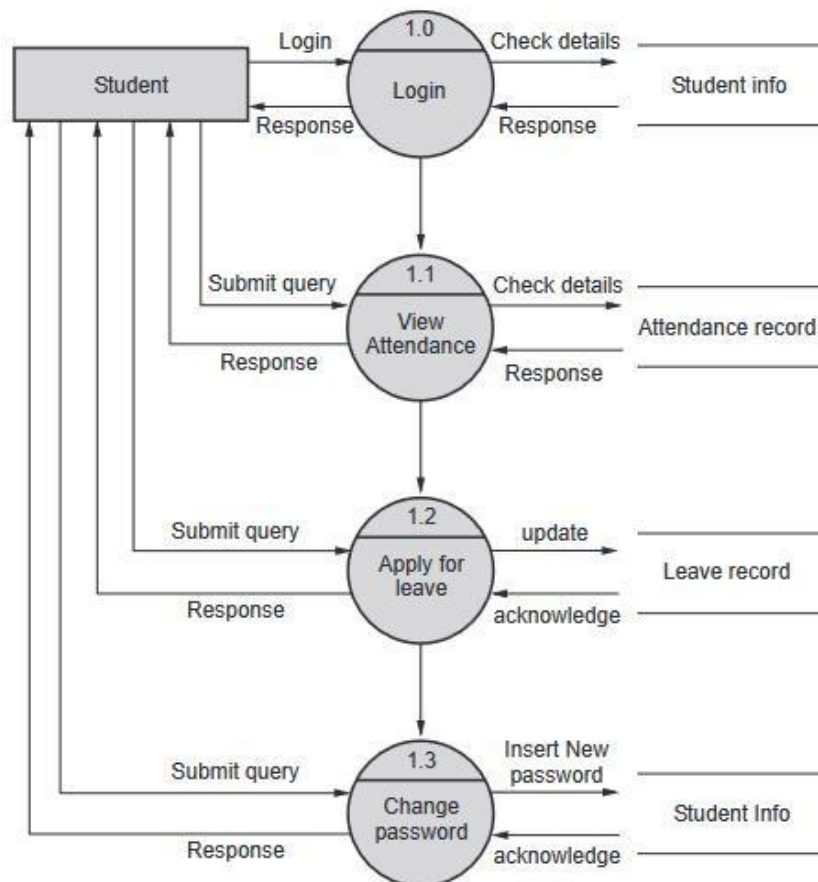
Fig. 2 Level 1 DFD
