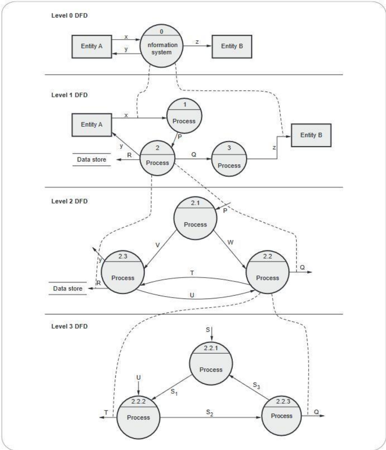
Fig. 3.4.1 Levels of DFD
